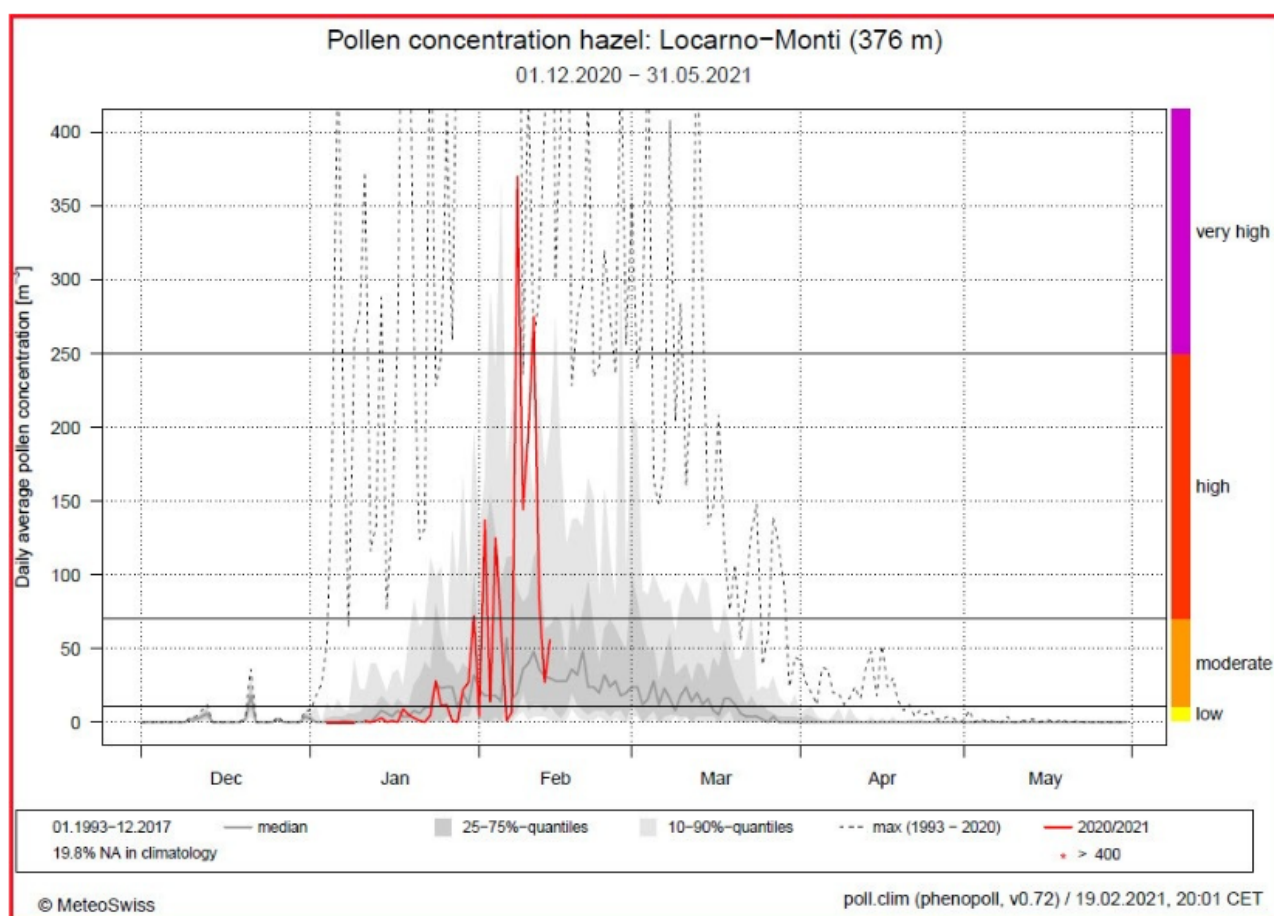
Fig. 2: Concentrazioni di polline di nocciolo rilevate a Locarno-Monti dal mese di dicembre 2020.
